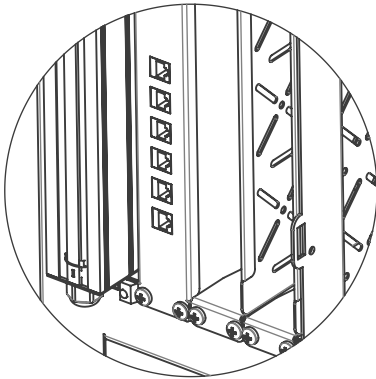
ВИД Р (1 : 5)
