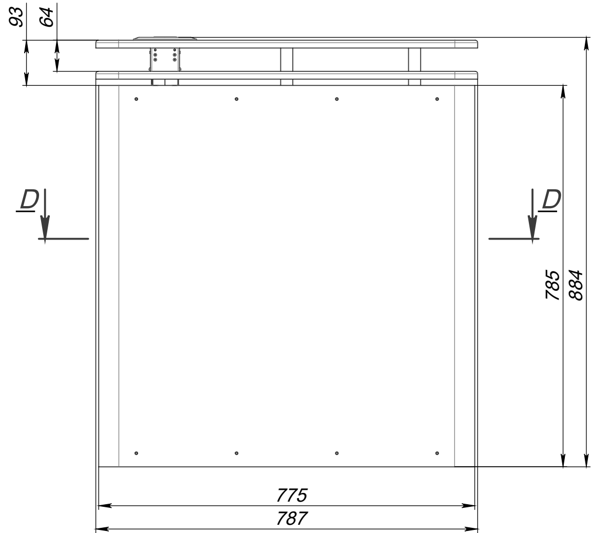
ВИД Р (1 : 5)
