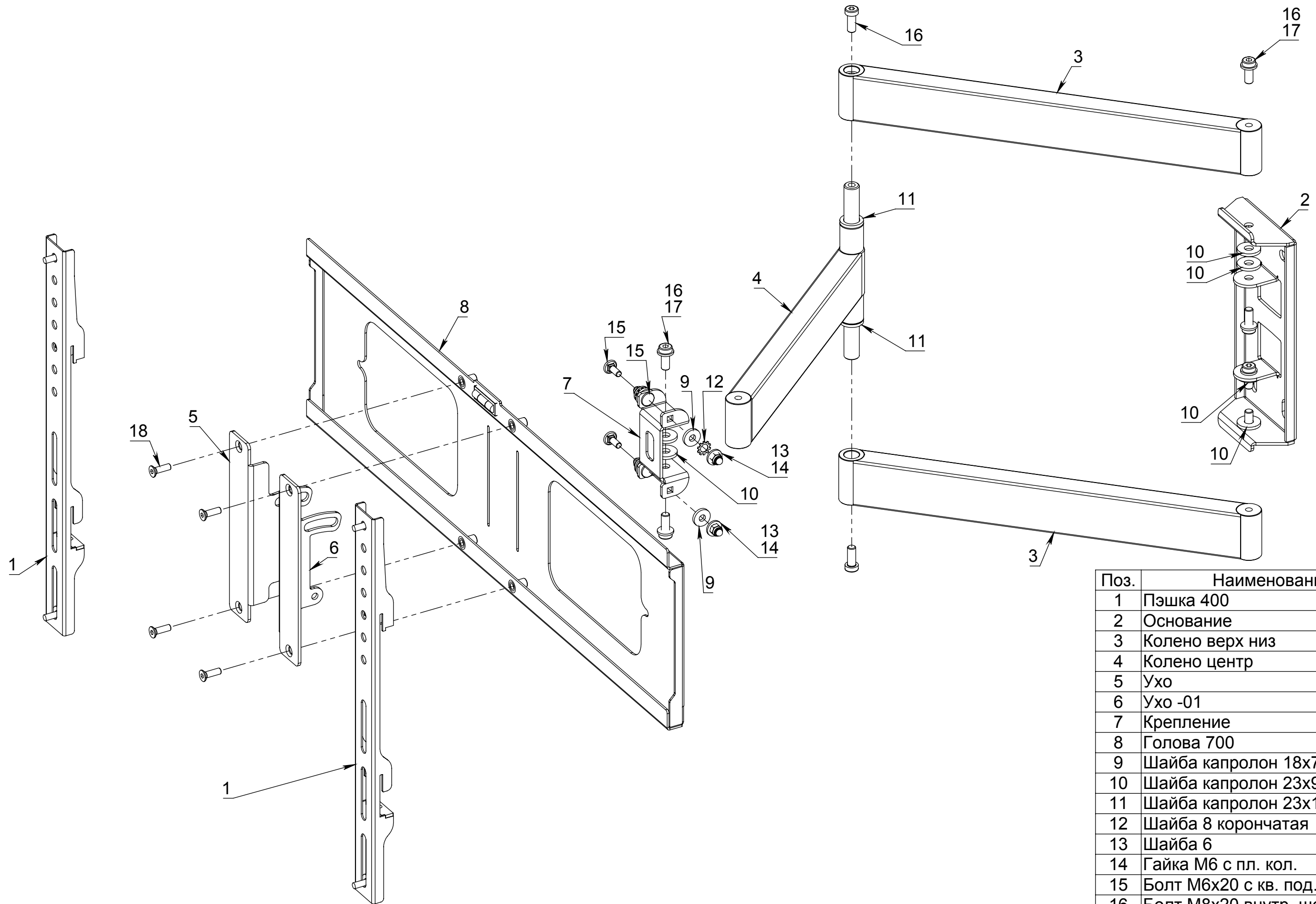
Крепление настенное для панели весом до 80 кг (крепеж 600x400)
