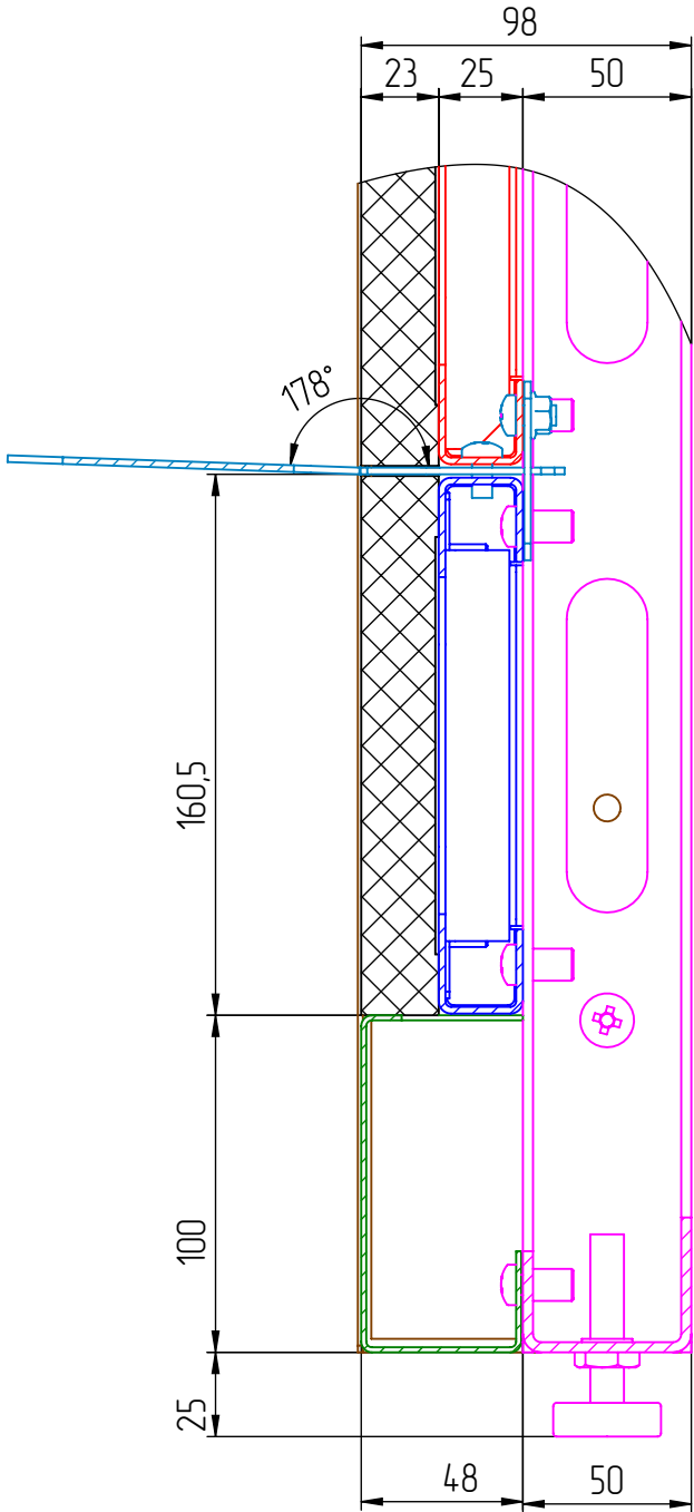
А2-А2 (1:10)
