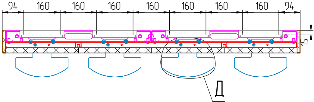
А2-А2 (1:10)
