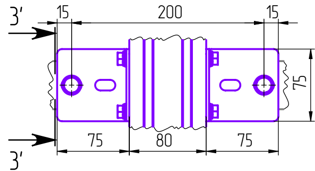
Узел крепления к перегородке. M1:4
