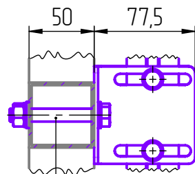
Болт M10x70 DIN 933 Гайка M10 DIN 934 Шайба 10 DIN 125 Шайба 10 DIN 7980
