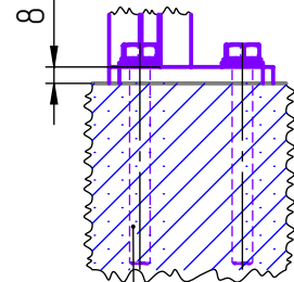
Анкер мунд Hilti HSA-F M10x83
