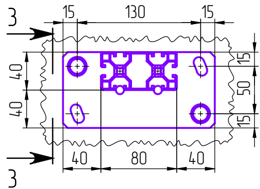
Узел крепления к полу. M1:4
