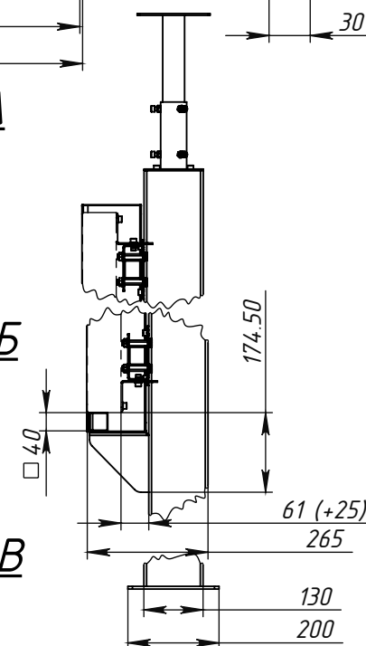
ВИД А
