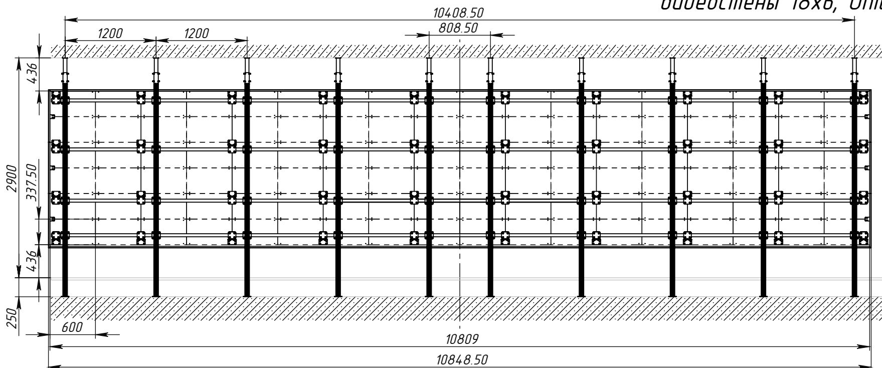
ВИД А
