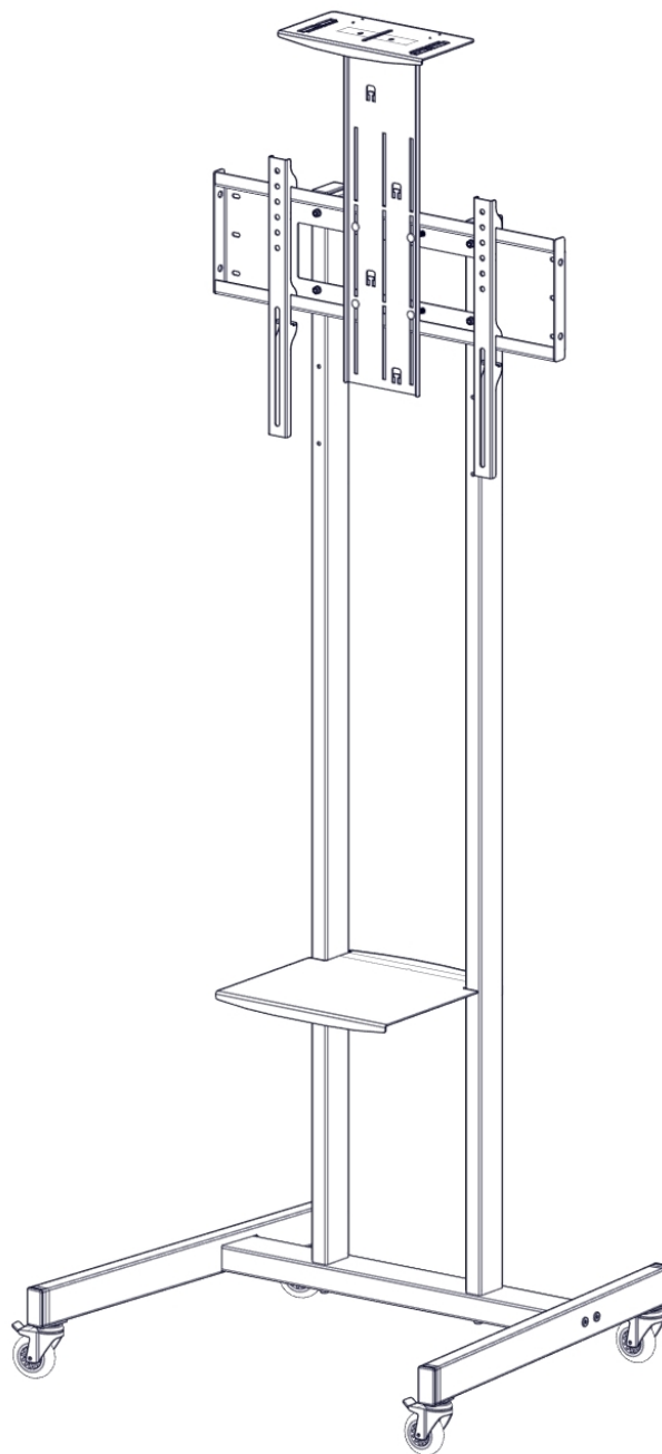
Рис. 1 – Стойка в сборе.
