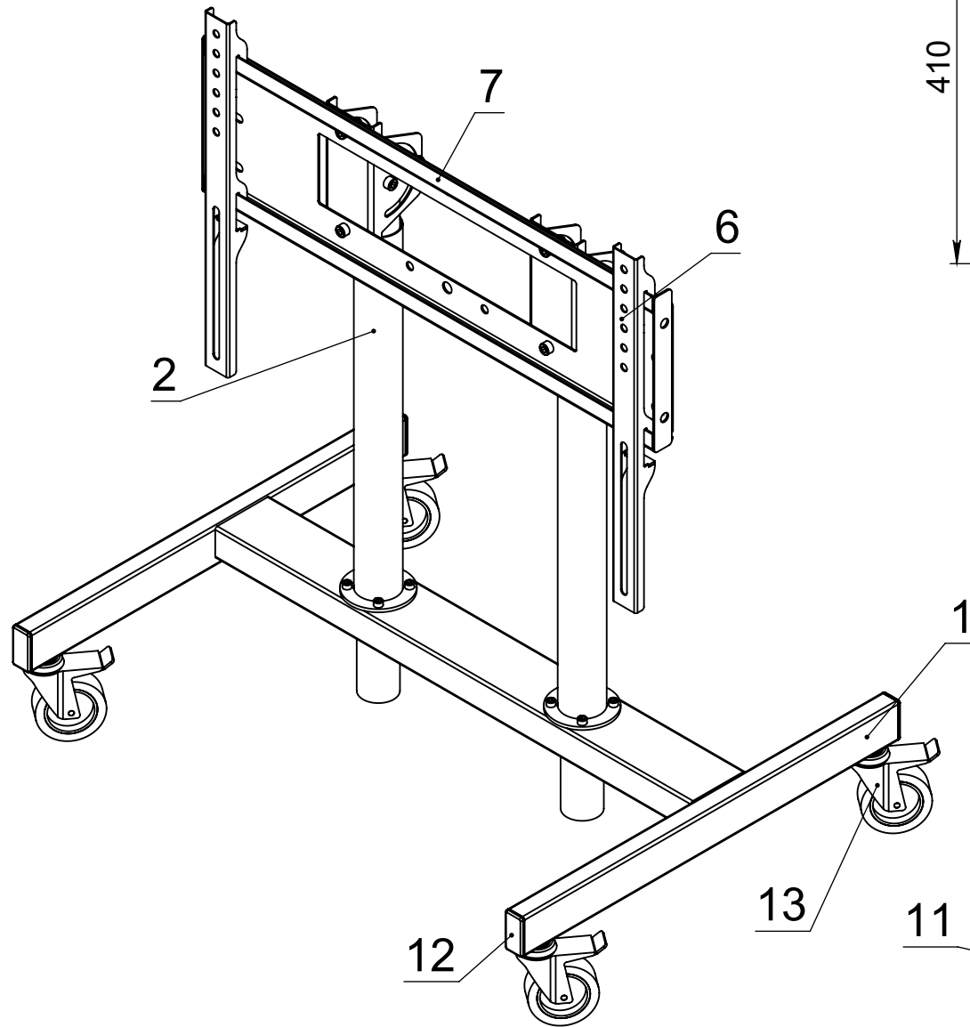
А (1 : 2)
