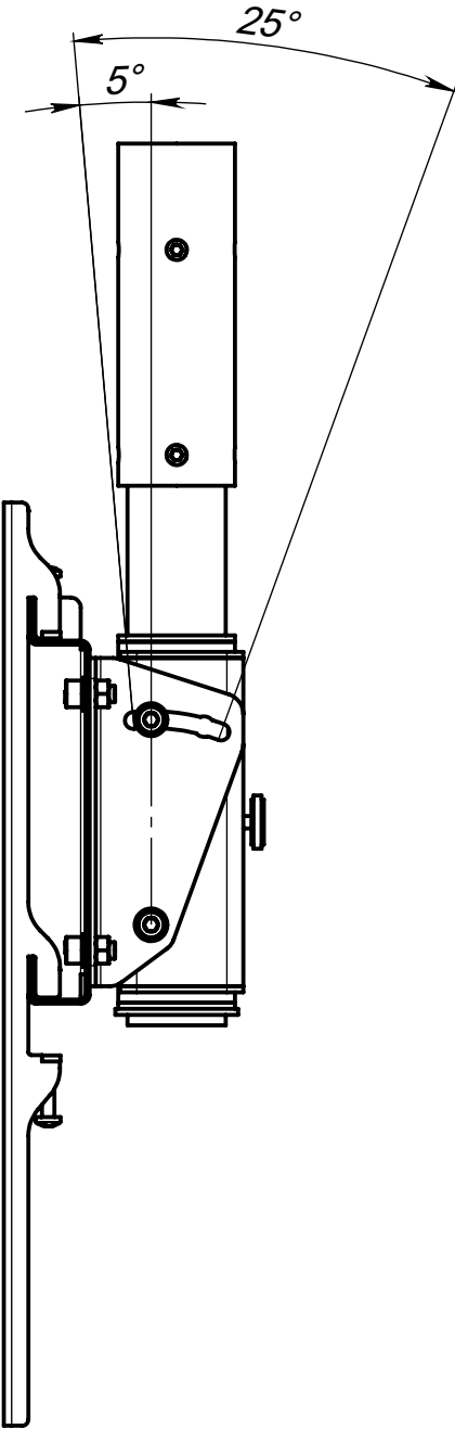
G-G (1 : 4)
