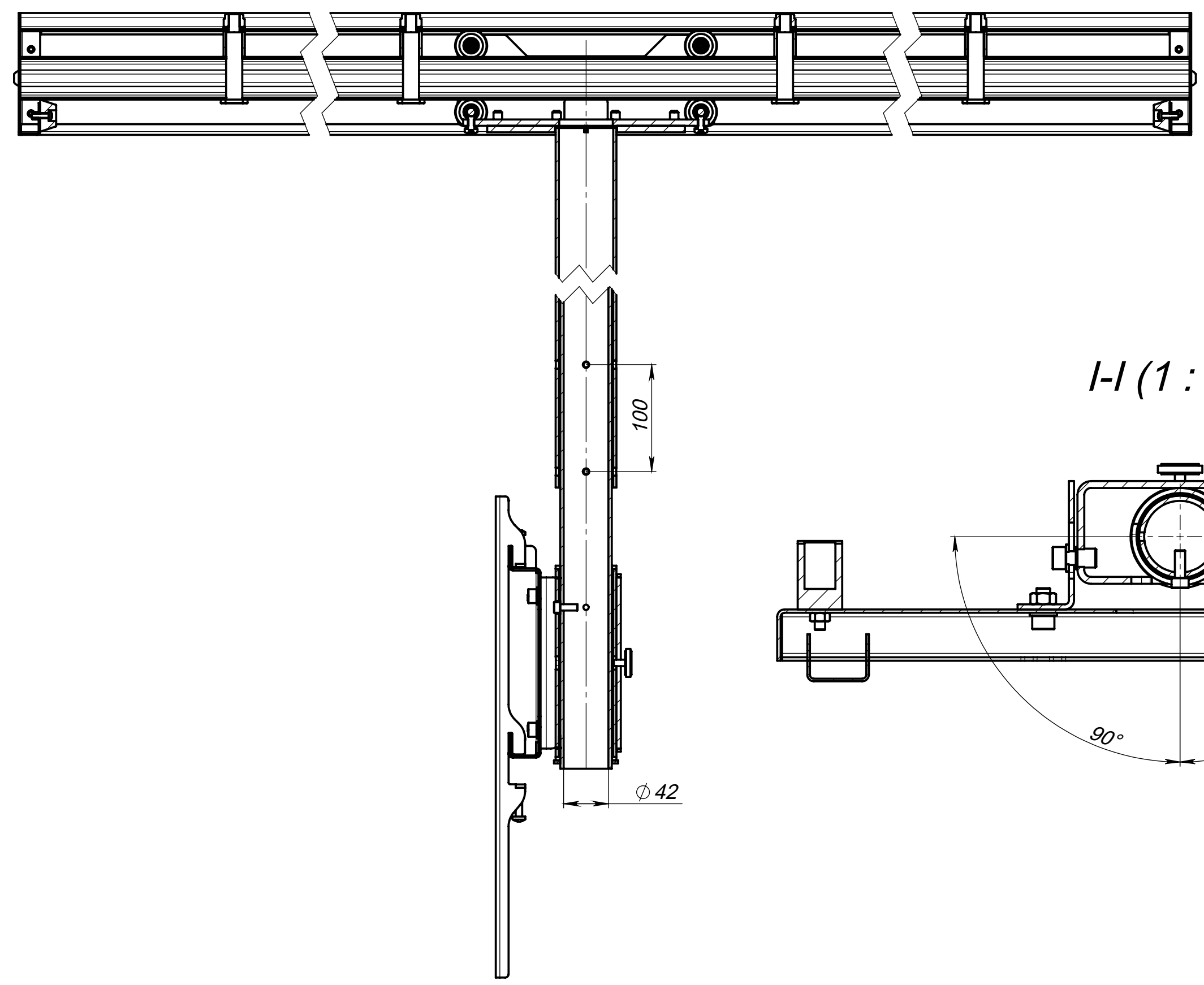
H-H (1 : 4)
