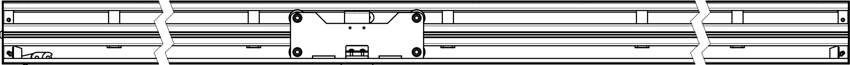
F-F (1 : 4)
