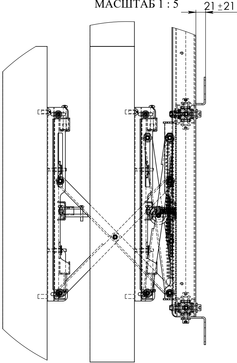
МЕСТНЫЙ В МАСШТАБ 1 : 5
