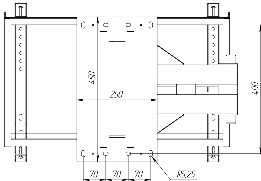
Вид сзади
