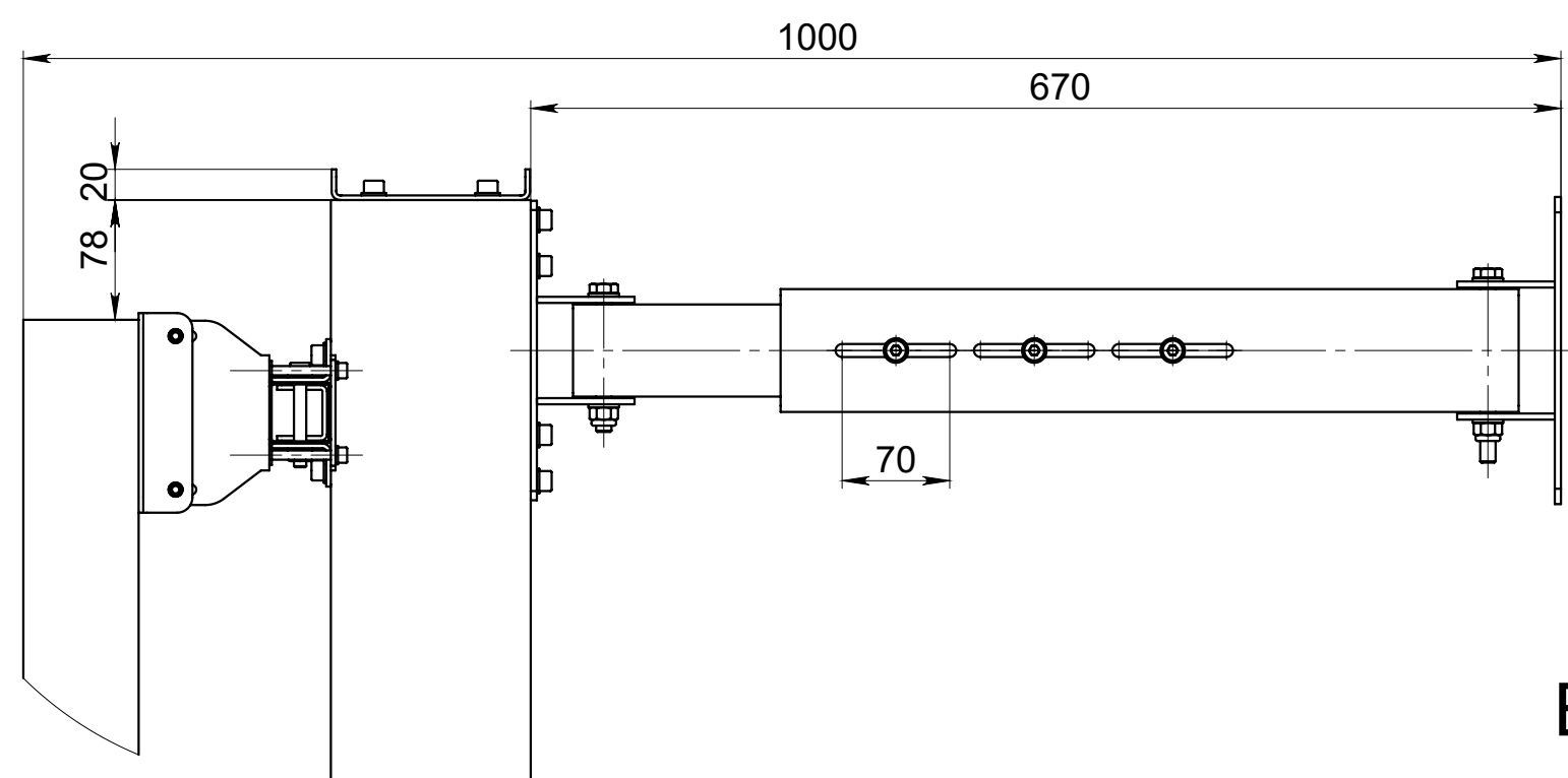
A (1 : 5)
