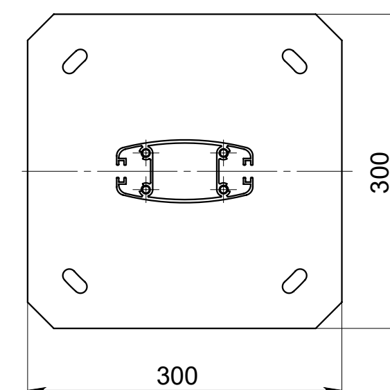
B-B (1 : 5)
