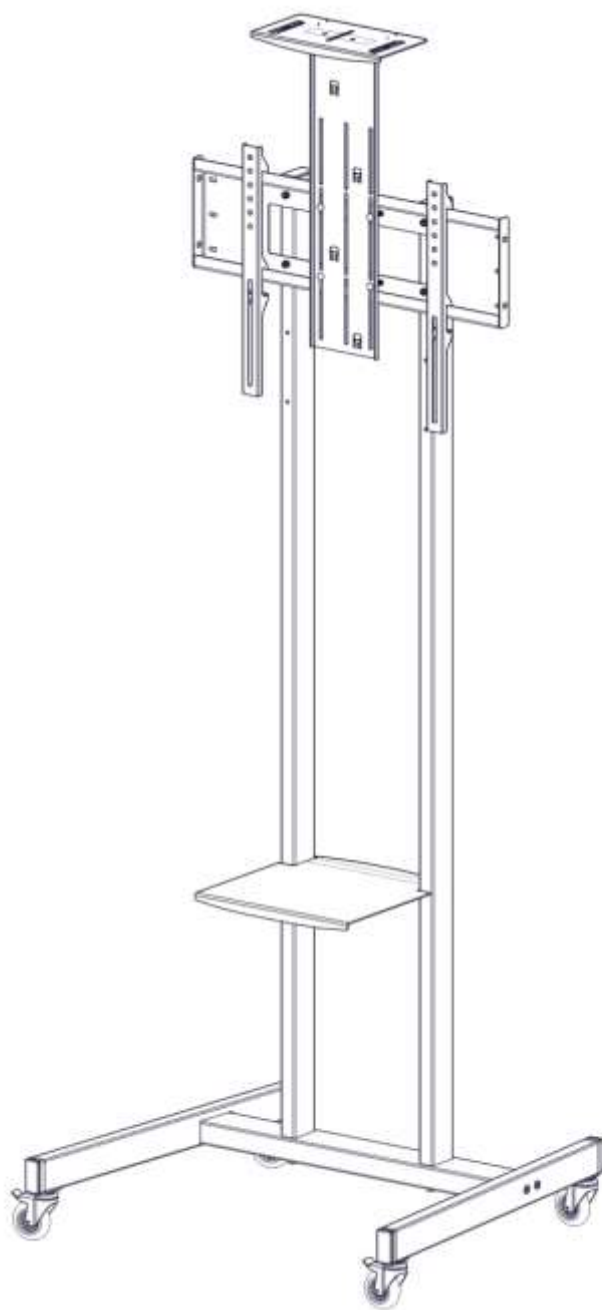
Рис. 1 – Стойка в сборе.
